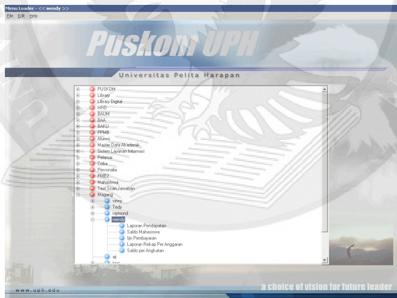
Gambar 4.3 Tampilan Menuloder
